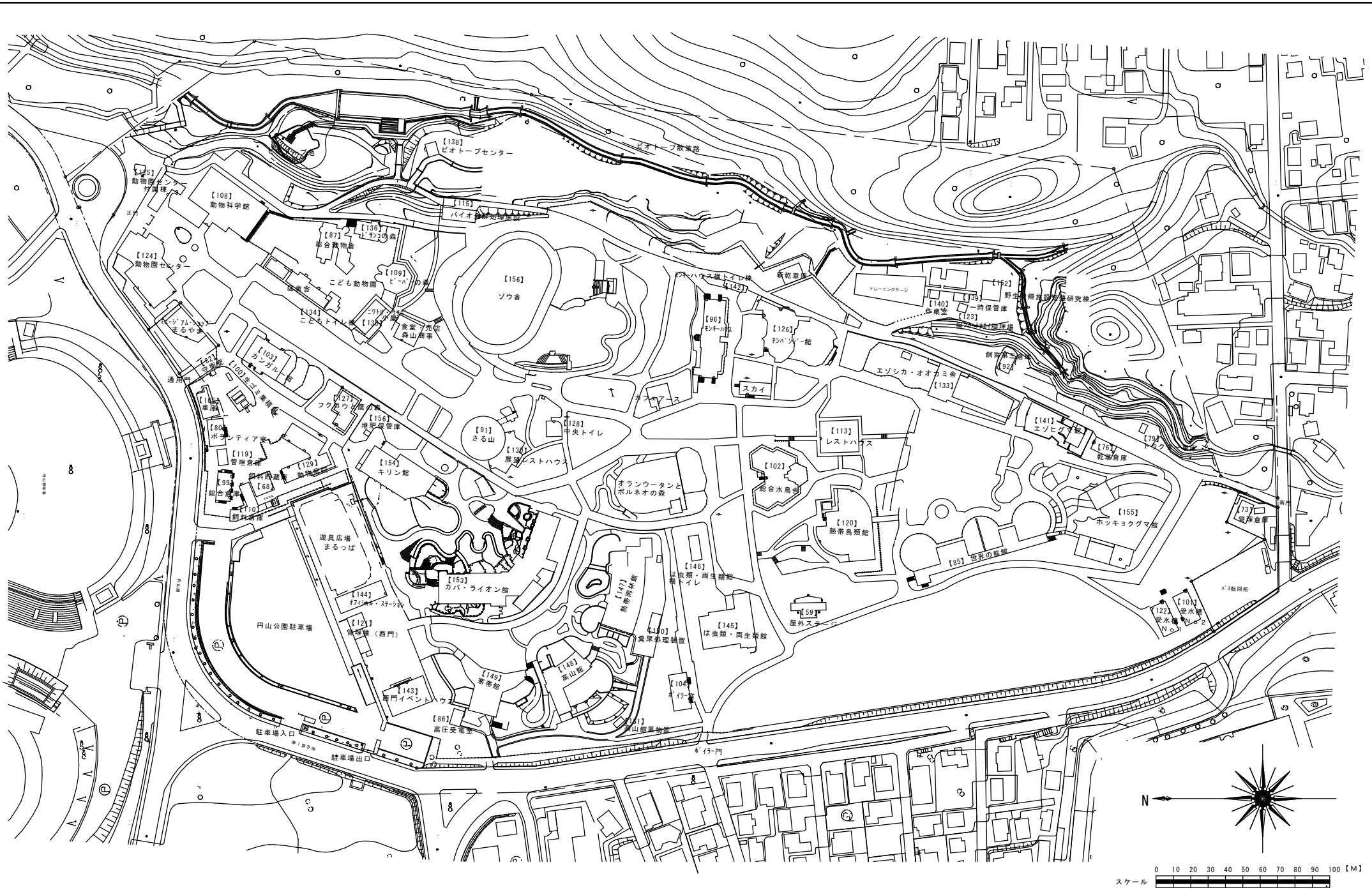
配置図 S=1/2,000 (A3)
