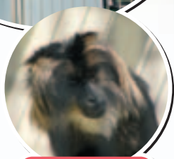
シシオザル
