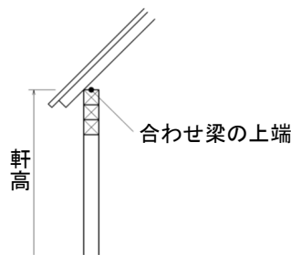
図2 木造（合わせ梁）
