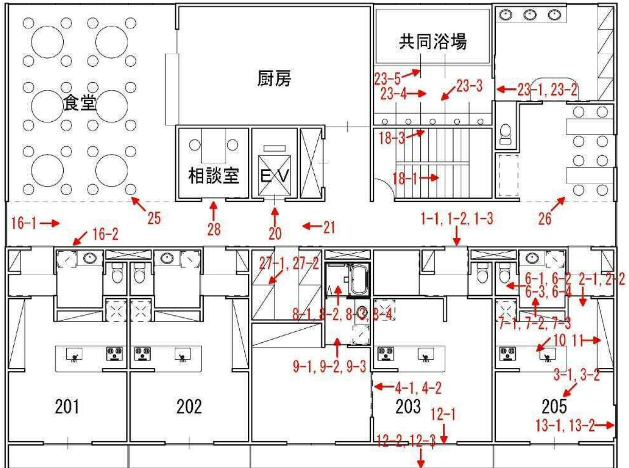
2階平面図
