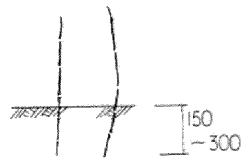
根入部寸法
