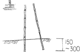
根入部寸法
