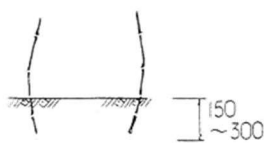
根入部寸法
