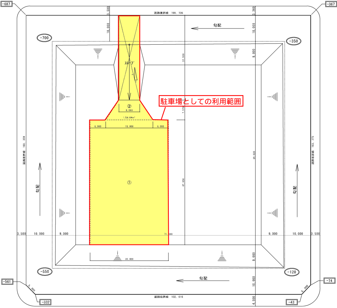
敷地造成図 1/300
