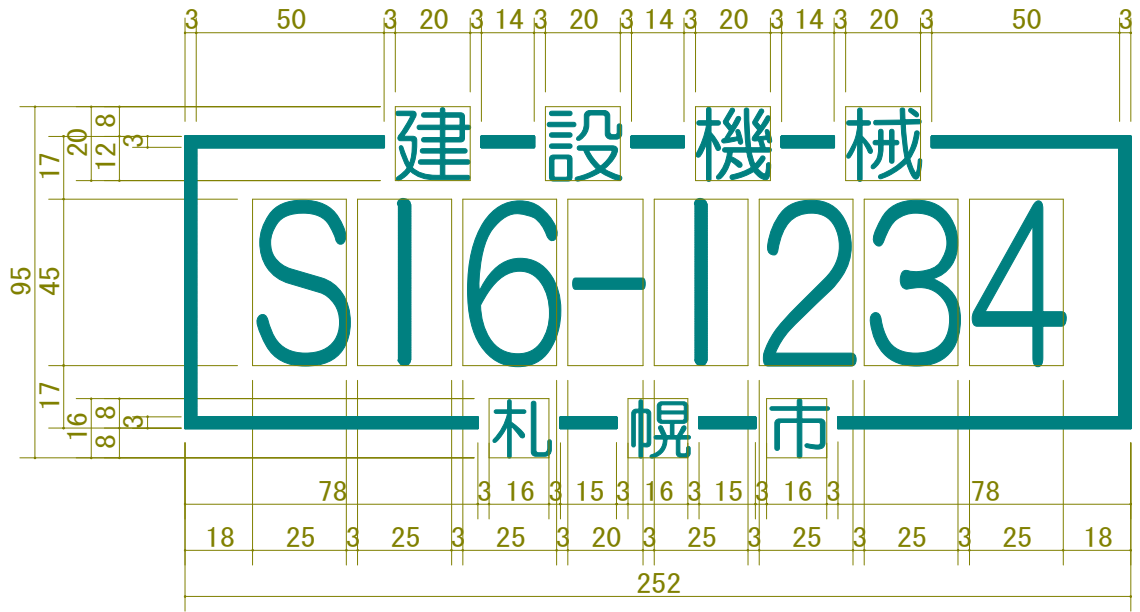
・別図—3 国土交通省補助除雪機械の表示例
