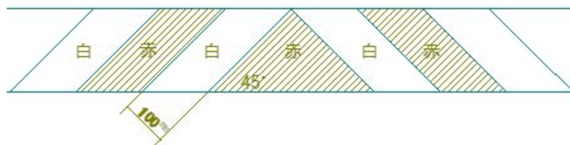
(ロ) 車両後部の赤白縞
