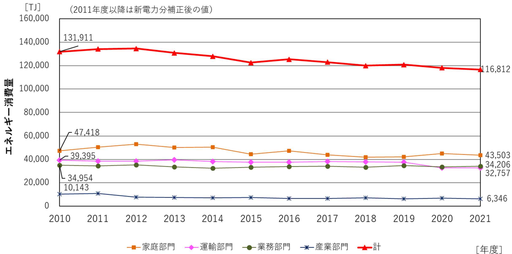
図 エネルギー消費量の部門別推移
