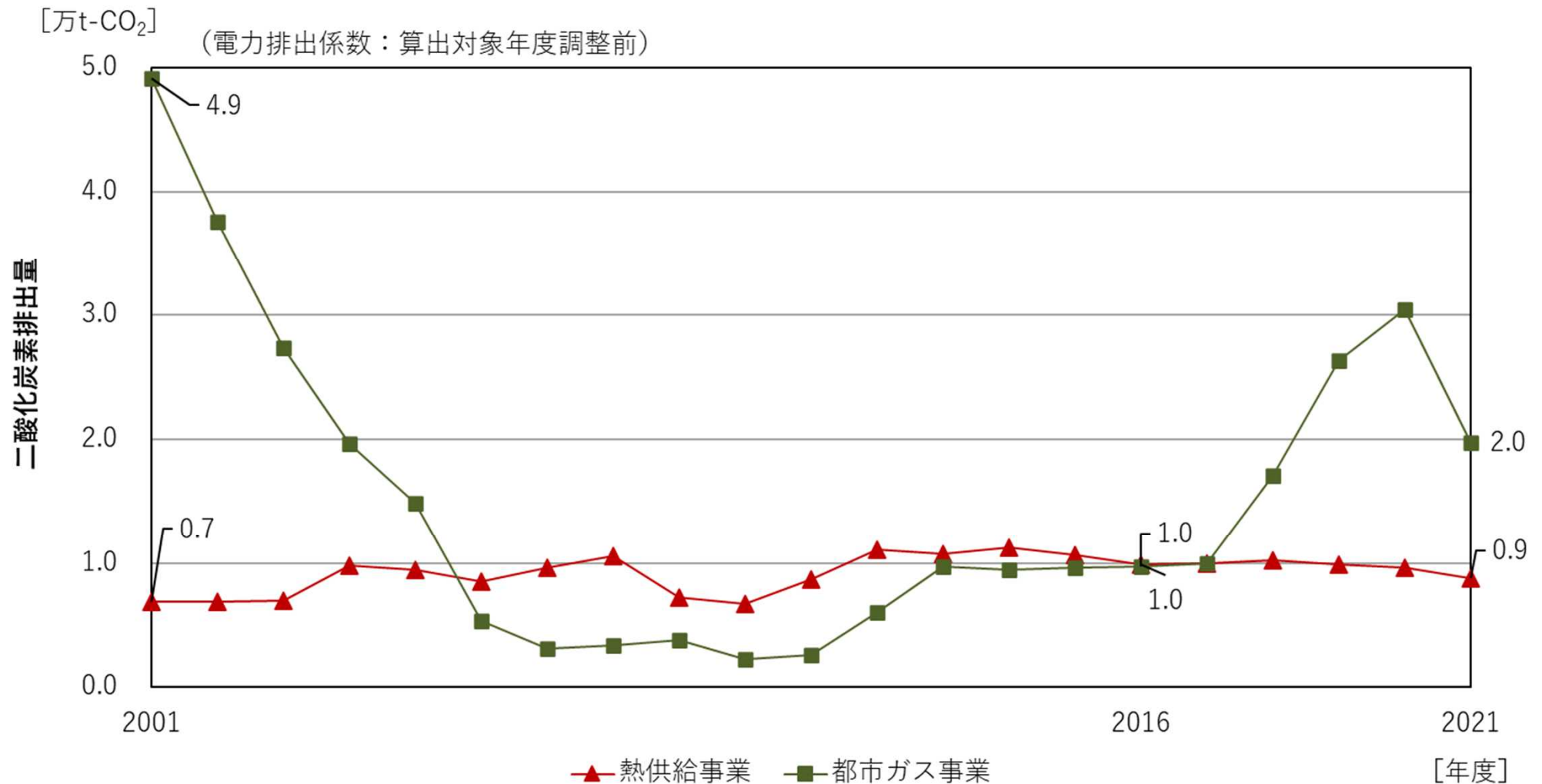
図 エネルギー転換部門の二酸化炭素排出量の事業別推移
