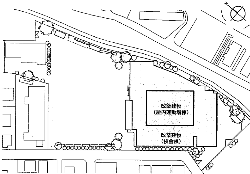
配置図
