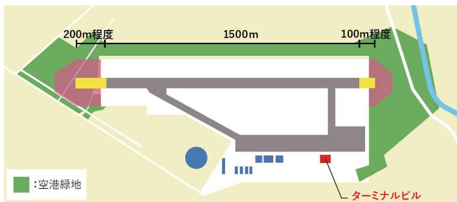
図7 滑走路長 1,800m とする場合のイメージ図
