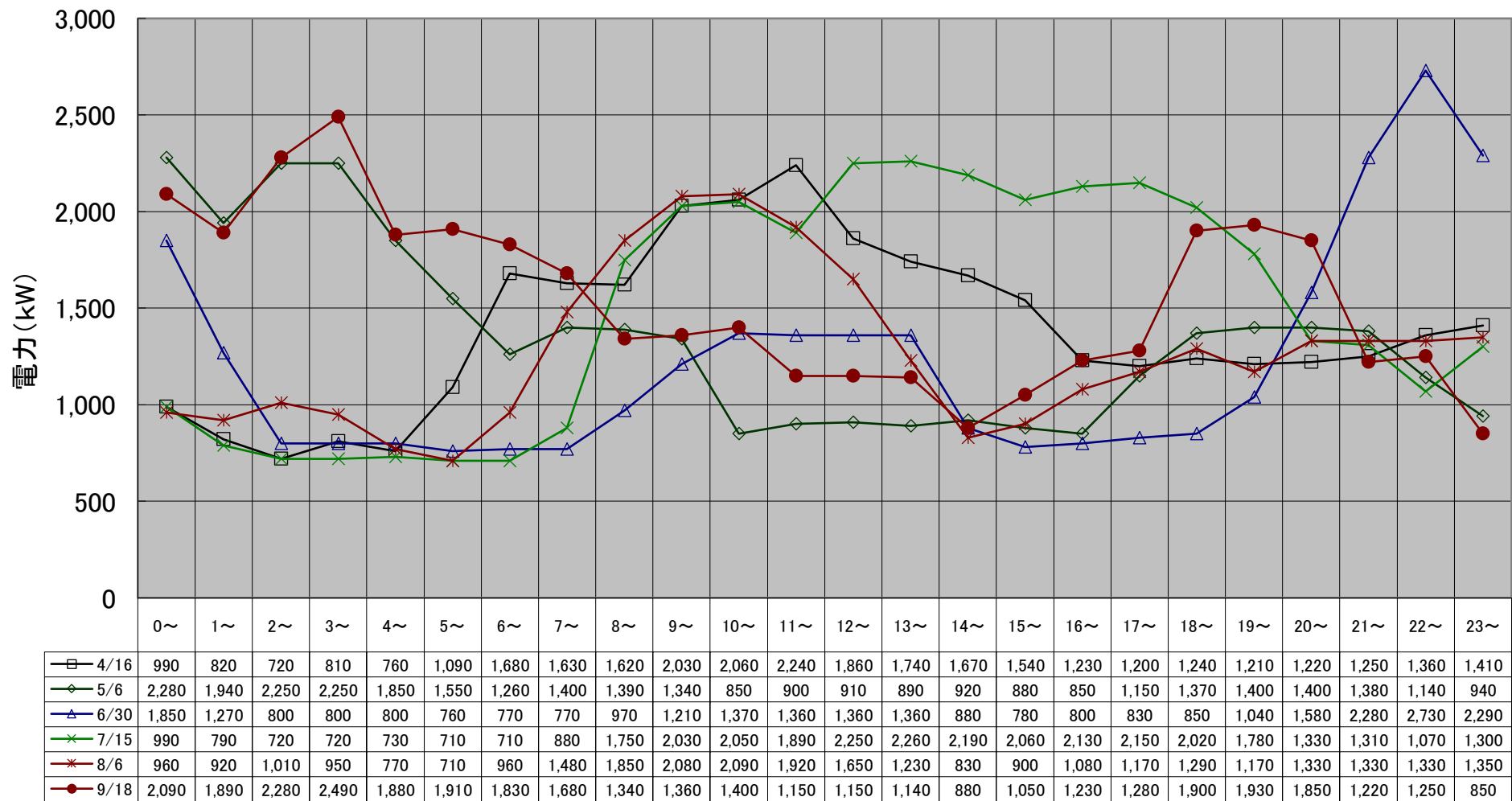
月別最大負荷日ロードカーブ(令和5年度上期)
