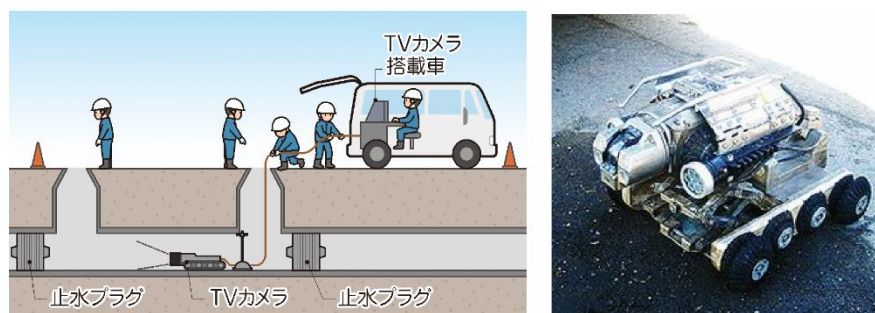
テレビカメラを用いた管路の詳細調査
